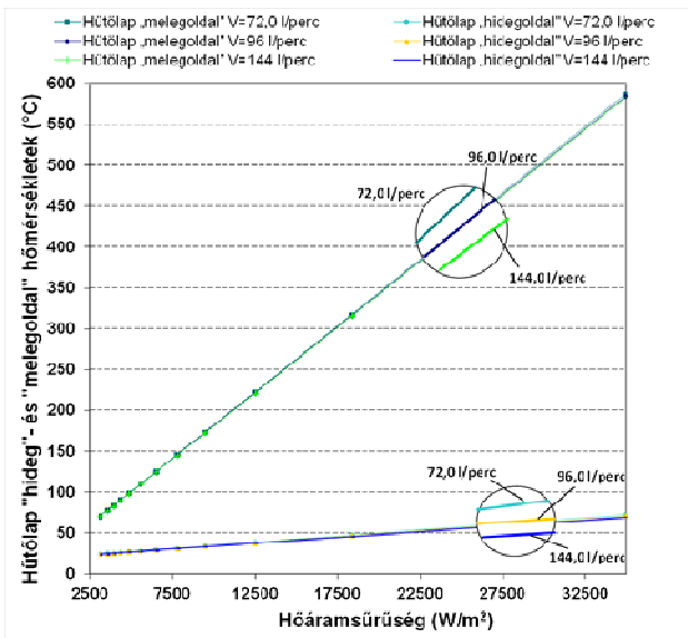
7. ábra A nagyolvasztó akna alsó részének hűtési modellel számított hűtőlap „meleg”- és „hidegoldali” hőmérsékleti értékek különböző hőáram-sűrűségek és hűtővíz-térfogatáramok mellett
